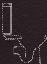
KOMBI WC S UNI ODPADOM
