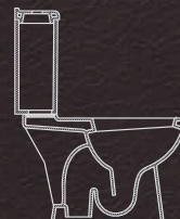
KOMBI WC SO SPODNÝM ODPADOM
